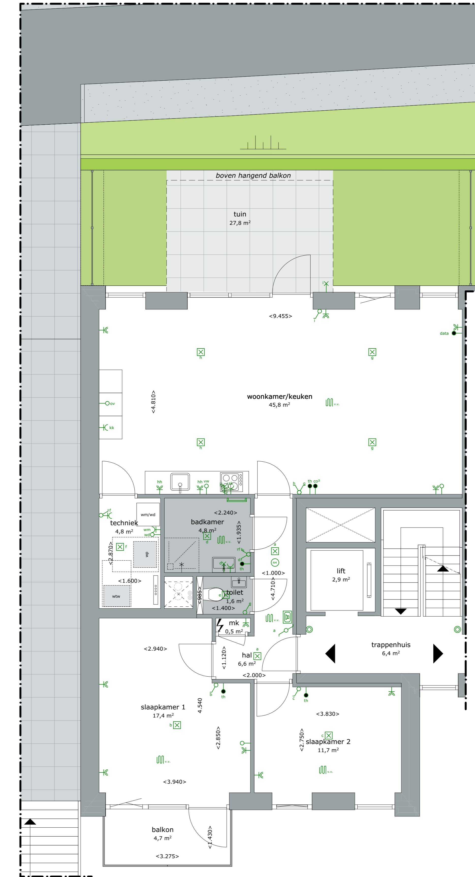
BEGANE GROND 1:50
