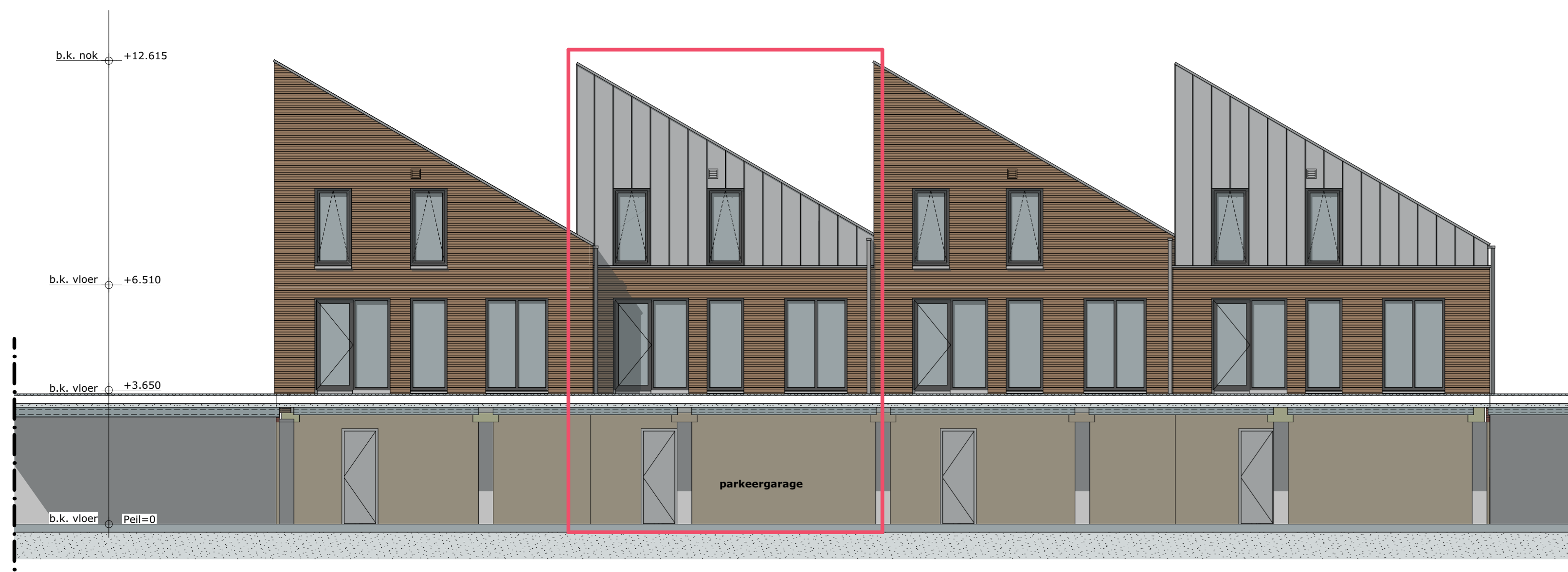
NOORDGEVEL C 1:100
