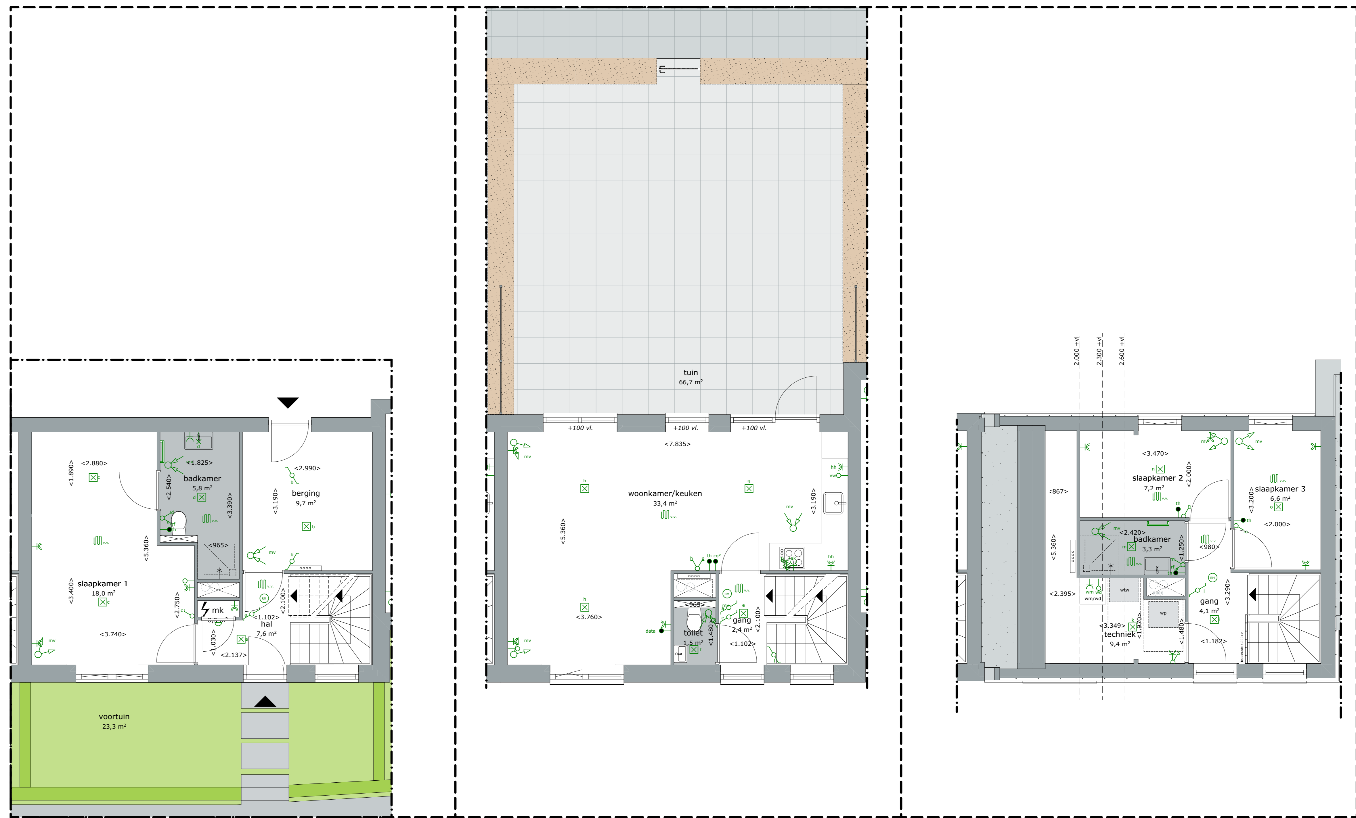
SOUTERRAIN 1:50
