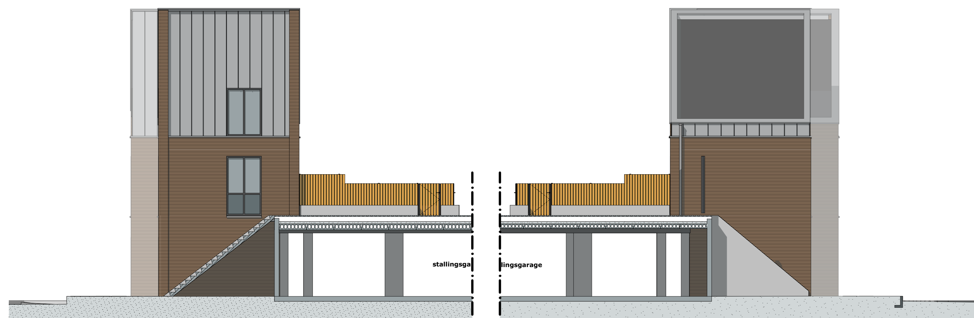
OOSTGEVEL C 1:100
