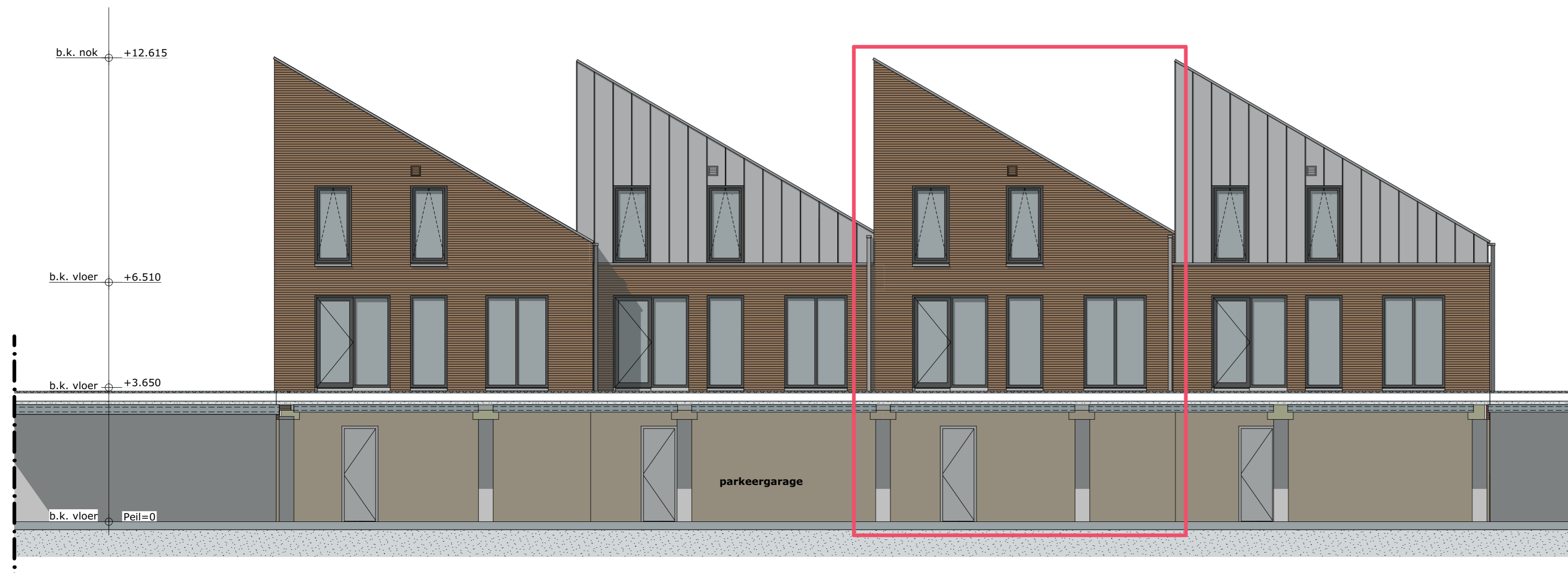
NOORDGEVEL C 1:100
